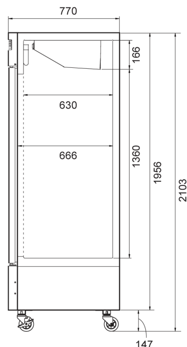
ВИД СБОКУ
