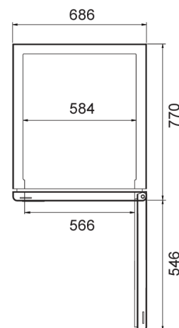
ВИД СВЕРХУ
