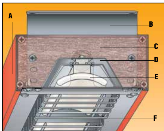
Схема UGA-60
